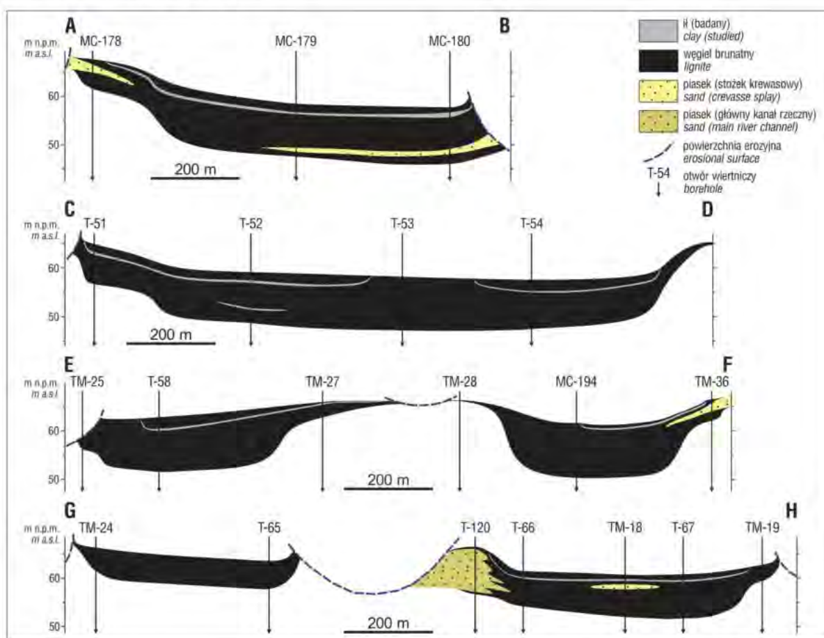
Ryc. 8. Uproszczone przekroje geologiczne ukazujące architekturę przewarstwień klastycznych (iłów i piasków) w obrębie pierwszego środkowopolskiego pokładu węglowego (środkowy miocen) w złożu Tomisławice. Lokalizacja linii przekrojowych na ryc. 3 Fig. 8. Simplified cross-sections depicting an architecture of the clastic interbeddings (clays and sands) within the first mid-Polish lignite seam in the Tomisławice deposit. For location of the cross-section lines see Fig. 3
